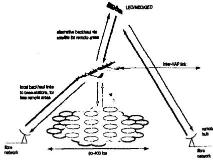
그림 1. HeliNet Network의 아키텍처 시나리오 Fig. 1. Scenario of HeliNet Network Architecture
