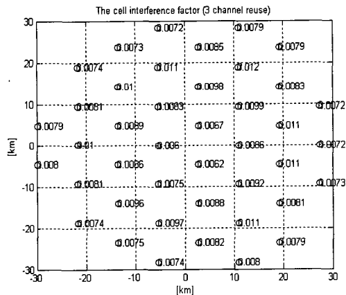
그림 6. 최적의 \theta_{3dB} 를 이용한 3 채널 주파수 재사용의 경우의 인접 셀 간섭계수에 대한 시뮬레이션
