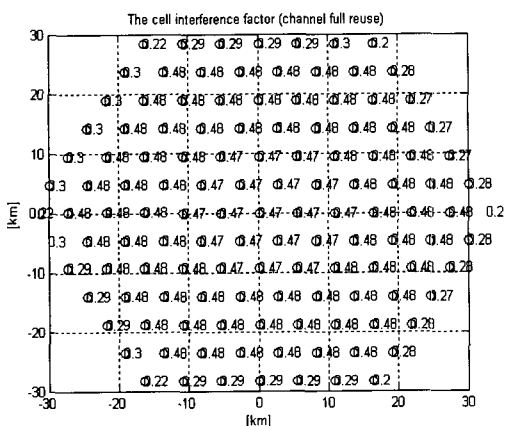
그림 5. 최적의 \theta_{3dB} 를 이용한 전채널 주파수 재사용의 경우의 인접 셀 간섭계수
