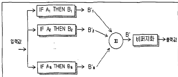
(그림 3) 퍼지 규칙 시스템 구현
