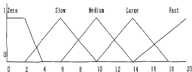
(그림 5) ①속도의 소속 함수
