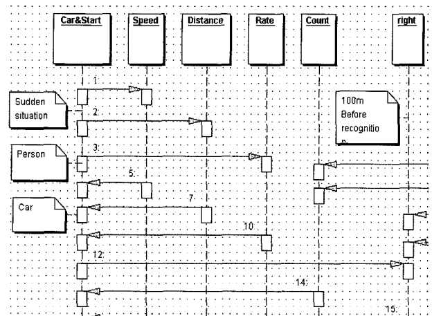
(그림 8) Sequence Diagram
