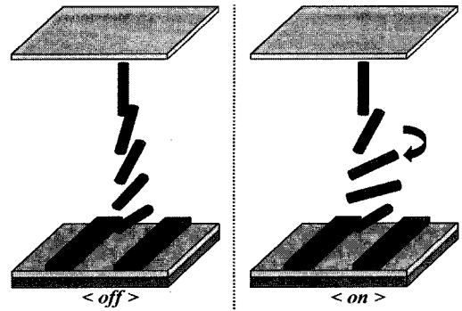
그림 1. 유전을 이방성이 양인 액정을 사용한 HAN-FFS 모드의 on-off 시의 액정 배열.
