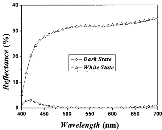
그림 5. 유전율이 이방성이 양인 액정을 이용한 반사형 HAN-FFS 모드에서 어둡 상태와 밝음 상태의 파장의존성.
