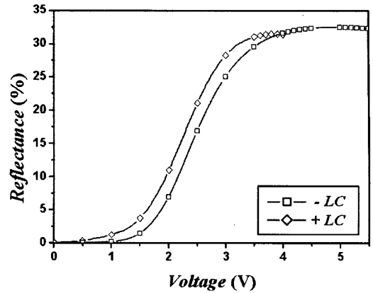
그림 4. 반사형 HAN-FFS 모드에서 입사 파장이 550 \text{nm} 에서 전압에 따른 반사율 곡선.
