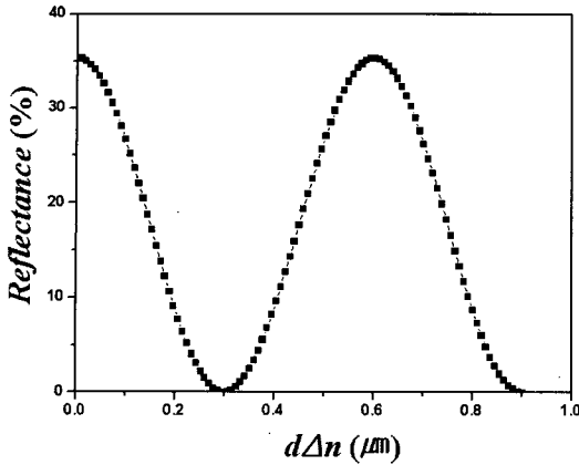
그림 3. 반사형 HAN-FFS 모드에서 어둡 상태에서의 d\Delta n 에 따른 반사율.
