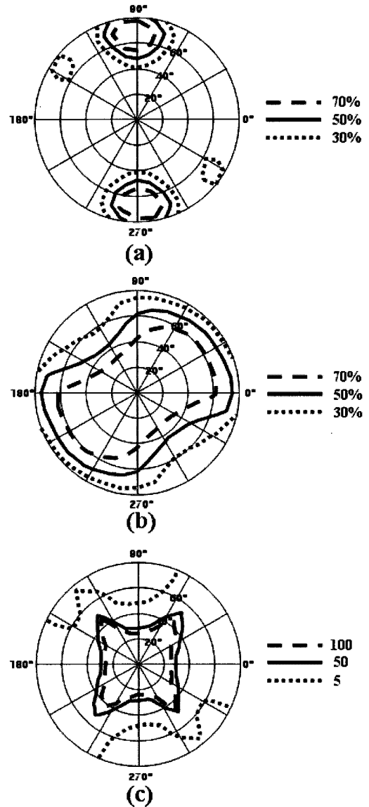
그림 6. 전과장 영역에서 어둡 상태 (a)와 밝음 상태 (b)의 등 휘도 곡선들과 등 명암 대비율 곡선(c).
