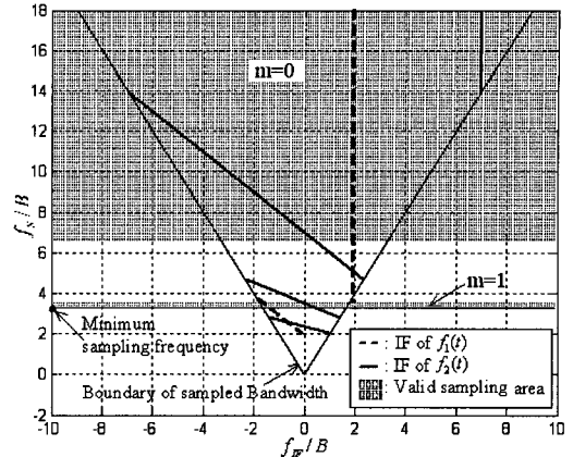
그림 10. Complex bandpass sampling 적용시 IF의 위치와 sampling 가능 영역
