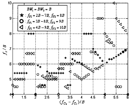
그림 11. Real bandpass sampling에 의해 요구되는 최소 sampling 주파수
