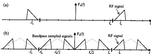
그림 2. (a) RF 신호, (b) Real bandpass sampling 방법에 의해 하향 변환된 신호들의 스펙트럼
