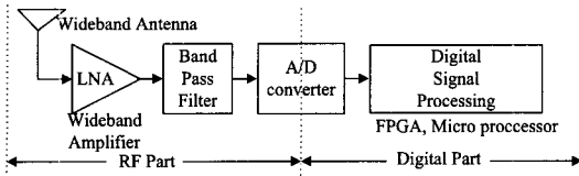
그림 1. SDR 수신기
