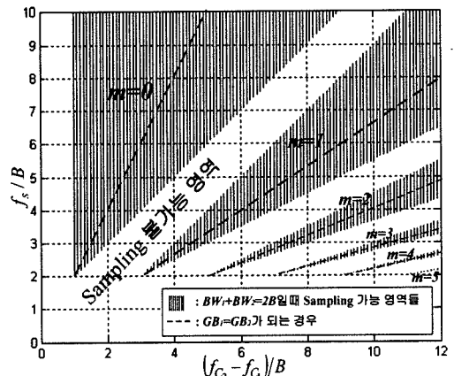
그림 5. Complex bandpass sampling에 의한 두 신호의 반송파 주파수 차와 sampling 주파수와의 관계
