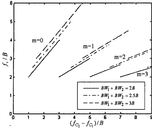
그림 12. Complex bandpass sampling에 요구되는 최소 sampling 주파수
