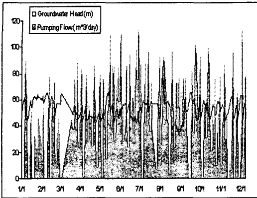
그림 2. 양수량에 따른 수위 변동 Figure 2. Water level change by flow quantity
