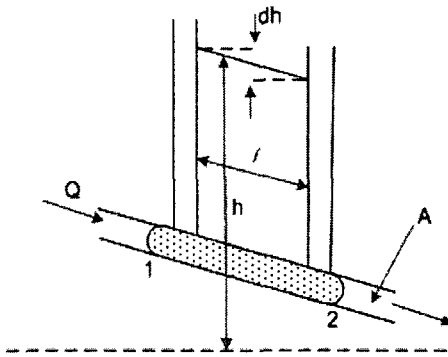
그림 1. Darcy의 법칙 Figure 1. Law of Darcy
