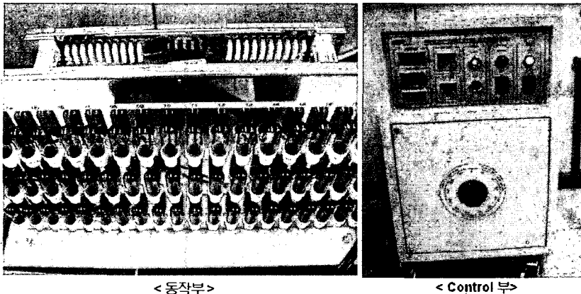
<그림 8> 가속수명시험장치 사진
