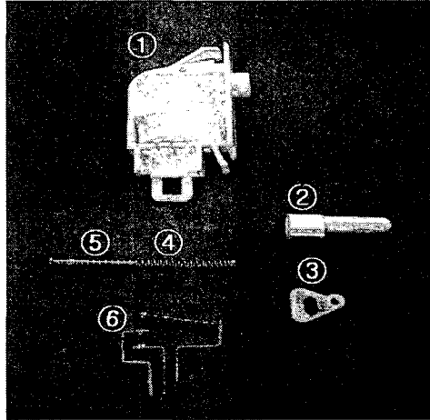
<그림 7> Architecture
