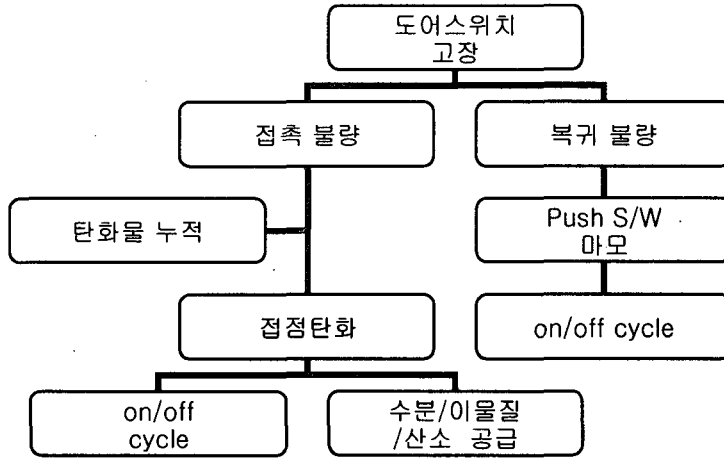
<그림 3> 도어스위치 조장모드/메커니즘
