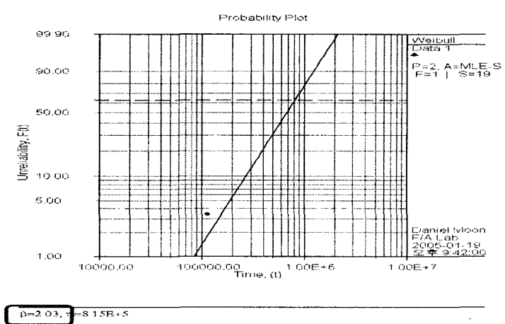
<그림 9> Weibull 분포도 (ALT)
