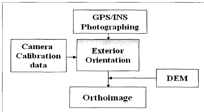
[그림 2] Direct Georeferencing에 의한 정사영상 생성 흐름도
