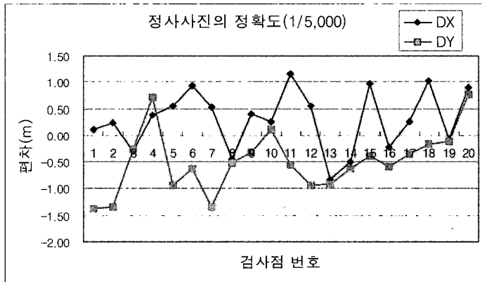
[그림 8] Direct Georeferencing 정사영상의 정확도
