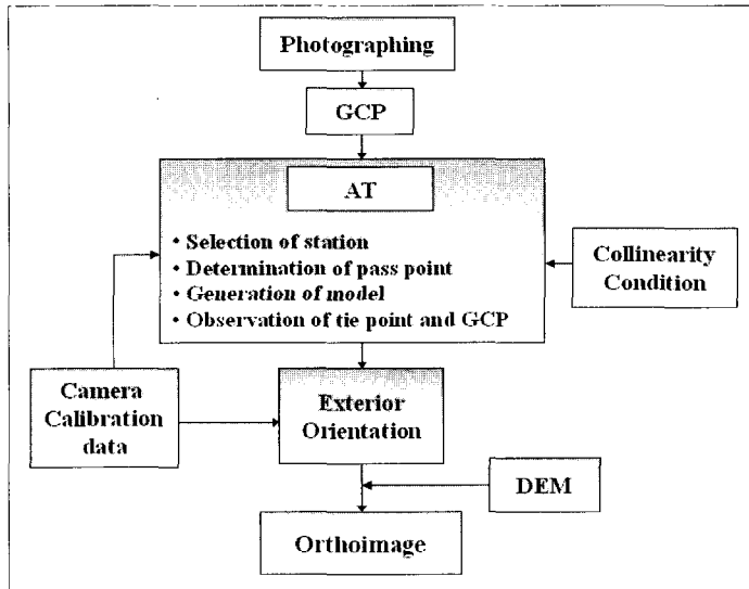
[그림 1] 기존 방법에 의한 정사영상 생성 흐름도
