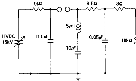
(a) 회로도
