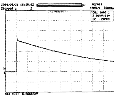
(b) 출력파형
