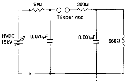
(a) 회로도
