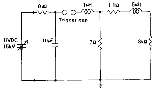
(a) 회로도
