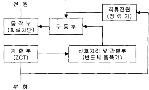
그림 1. 누전차단기의 구성 Fig 1. Configuration of an ELBs.
