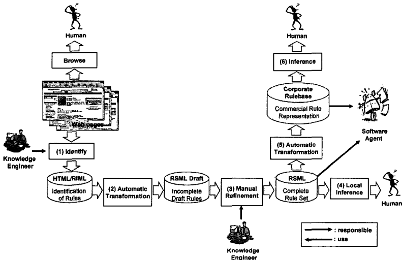
<그림 1> XRML을 이용한 규칙습득 과정
