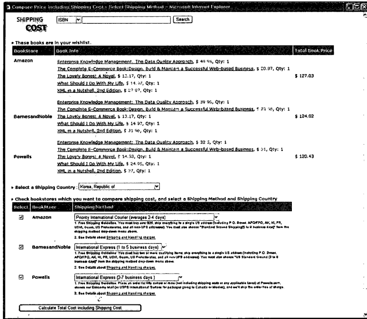
[그림 7] ConsiderD의 배송방법선택 화면의 예
