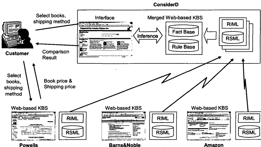
[그림 5] ConsiderD의 구조도
