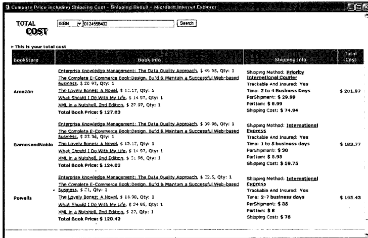
[그림 8] 배송비가 포함된 비교 결과화면의 예
