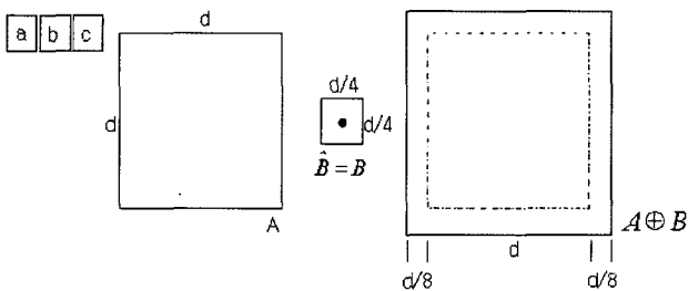
(그림 2) 팽창 연산
