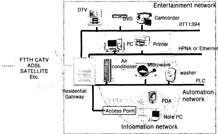
(그림 1) 홈네트워킹의 한 예
