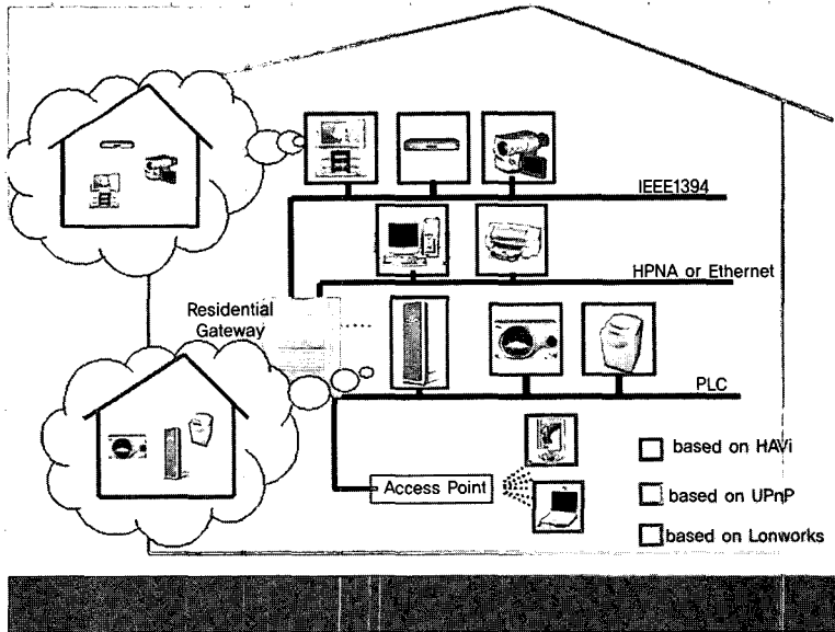
(그림 2) 홈 네트워킹 구성사례
