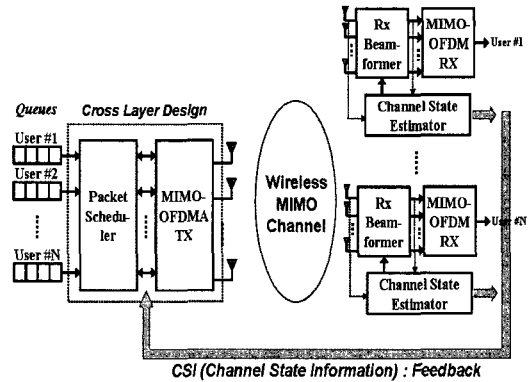
그림 1. MIMO-OFDM 다중 사용자 시스템 구조
