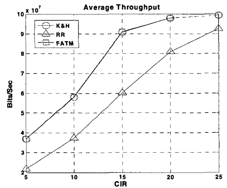
그림 5. CIR의 변화에 따른 스케줄링 방식별 평균 시스템 전송효율
