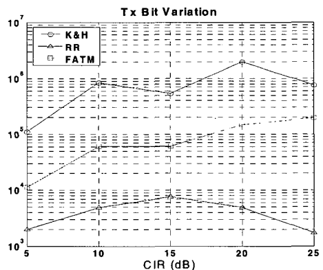
그림 6. 채널 상태 변화에 따른 스케줄링 방식별 전송 비트의 분산값
