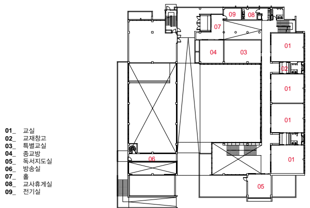
2층 평면도(유치원)
