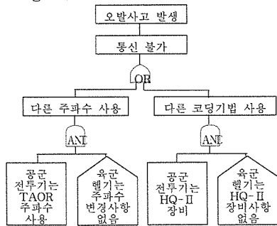
Fig.4 예제의 고장수목도(Fault Tree)
