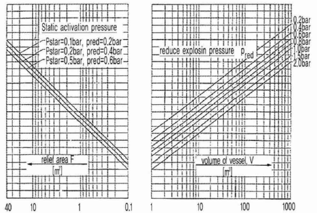
[도표 1] 메탄, 천연가스의 계산도표 (K G =bar · m · s -1 , 약한 발화원, 난류 없음)
