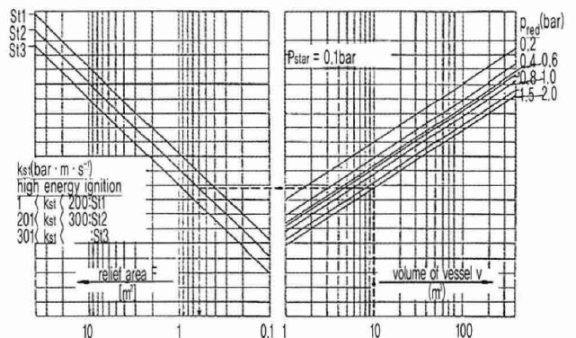
[도표 2] P Star =0.1 bar인 분진의 계산도표
