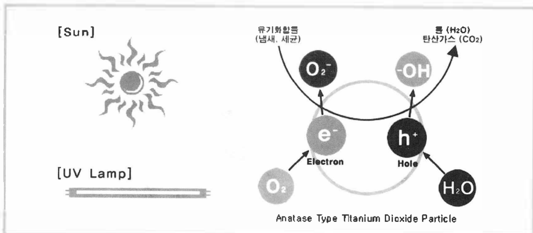
그림1. 광촉매 이산화티타늄의 산화분해 반응경로
