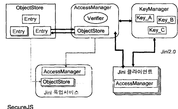
(그림 3) SecureJS 시스템의 구조
