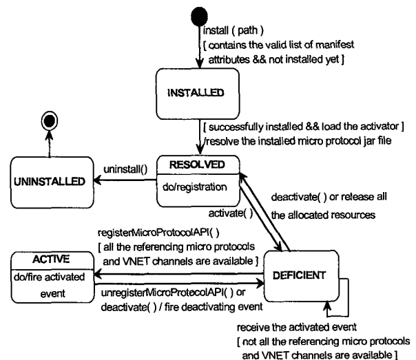
(그림 5) 마이크로 프로토콜 상태 전이도
