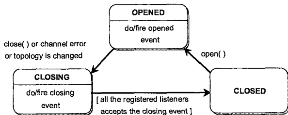
(그림 4) 가상 네트워크 채널 상태 전이도
