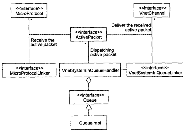
(그림 9) 액티브 패킷 수신 방법
