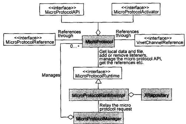
(그림 10) 마이크로 프로토콜 런타임 환경
