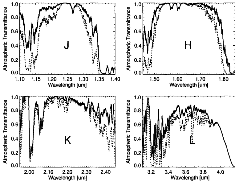
그림 3. 계산된 이산화탄소 상공의 대기 투과율(J, H, K, L 밴드, 천정거리는 60도). 겨울(PWV = 5.0mm - 실선)과 여름(PWV = 33mm - 점선).
