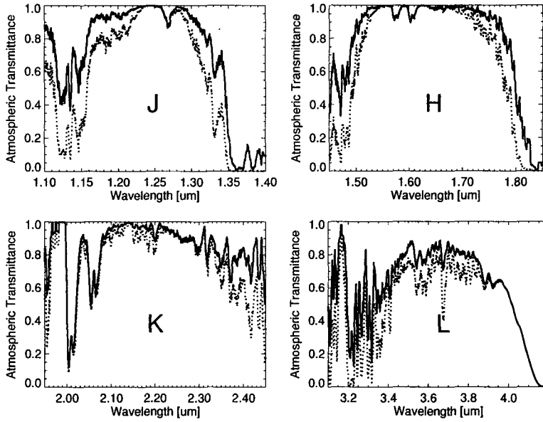
그림 2. 계산된 이산화황 상공의 대기 투과율(J, H, K, L 밴드, 천정거리는 60도). 겨울(PWV = 4.2mm - 실선)과 여름(PWV = 25mm - 점선).
