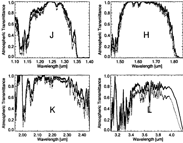
그림 6. 천정거리에 따른 대기 투과율 차이(J, H, K, L 밴드). PWV = 33mm, 천정거리 0도(실선), 60도(점선).
