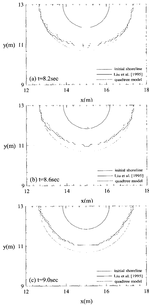
그림 7. 원형섬 전면에서의 범람영역
