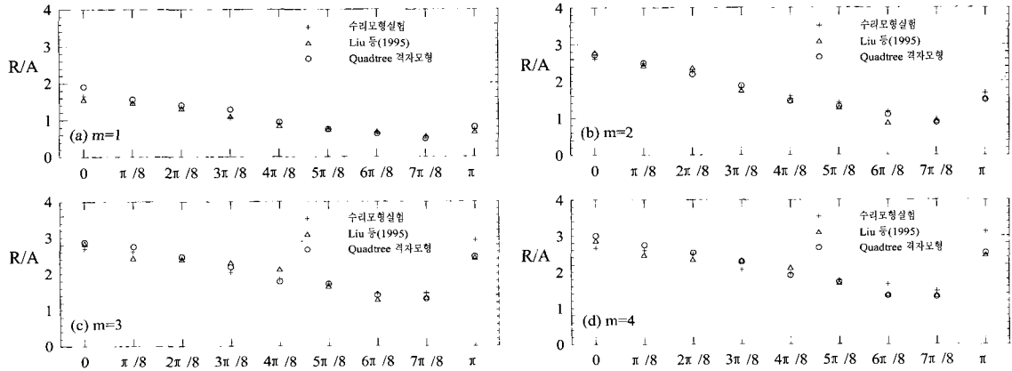
그림 6. 원형섬 주변에서의 최대 처오름높이 비교
