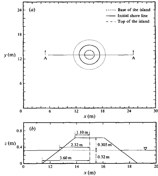
(a) 평면도 (b) 원형섬의 단면도 그림 2. 수리모형실험 장치:
