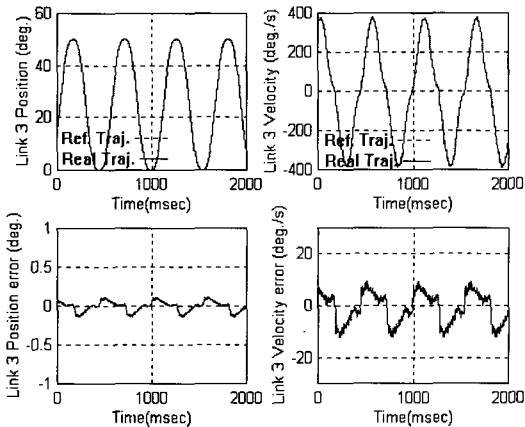
그림 16. 자기구성 퍼지제어기에 의한 링크3의 위치 및 속도 궤적 추종 결과. Fig. 16. The experimental results of SOFC for position and velocity trajectory tracking of link 3.(2.0kg payload).
