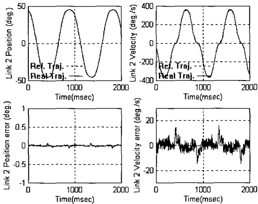
그림 15. 자기구성 퍼지제어기에 의한 링크2의 위치 및 속도 궤적 추종 결과. Fig. 15. The experimental results of SOFC for position and velocity trajectory tracking of link 2.(2.0kg payload).
