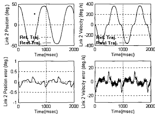
그림 19. PID제어기에 의한 링크2의 위치 및 속도 궤적 추종 결과. Fig. 19. The experimental results of PID controller for position and velocity trajectory tracking of link 2.(2.0kg payload).
