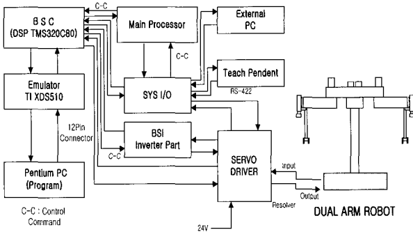
그림 12. 제어시스템의 구성도. Fig. 12. The block diagram of control system.
