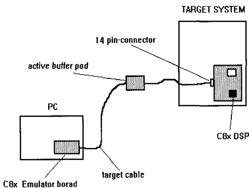
그림 13. 에뮬레이터 및 타겟 시스템의 셋업. Fig. 13. Equipment setup using the emulator and target system.
