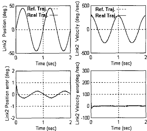
그림 8. 링크2의 위치와 속도 궤적 추종 결과. Fig. 8. Simulation results of position and velocity trajectory tracking for link 2.(2kg payload).
