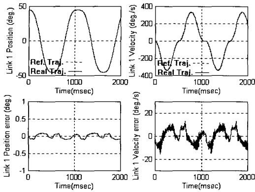
그림 14. 자기구성 퍼지제어기에 의한 링크1의 위치 및 속도 궤적 추종. Fig. 14. The experimental results of SOFC for position and velocity trajectory tracking of link 1.(2.0kg payload).
