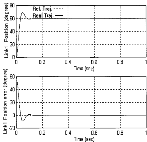
그림 5. 링크1의 위치궤적 추종 결과.
