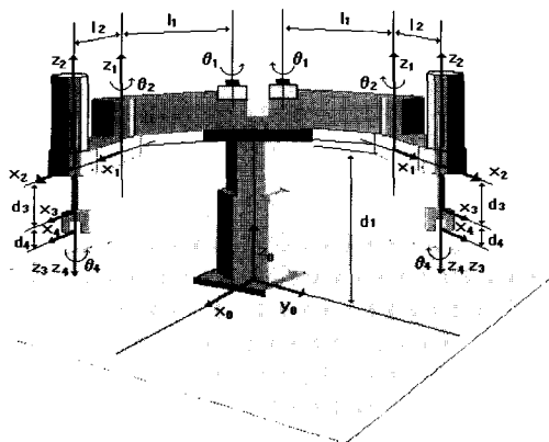
그림 3. 8축아암 로봇의 자표계 구조 Fig. 3. Coordinate frame of dual-arm robot with eight joints.
