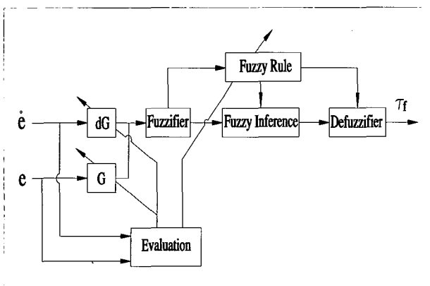
그림 1. 퍼지제어기의 구성도.
