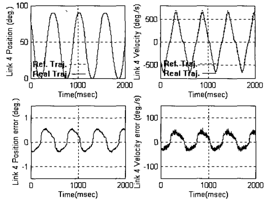
그림 17. 자기구성 퍼지제어기에 의한 링크4의 위치 및 속도 궤적 추종 결과. Fig. 17. The experimental results of SOFC for position and velocity trajectory tracking of link 4.(2.0kg payload).
