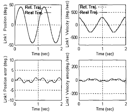
그림 9. 링크1의 위치와 속도 궤적 추종 결과. Fig. 9. Simulation results of position and velocity trajectory tracking for link 1.(2kg payload).
