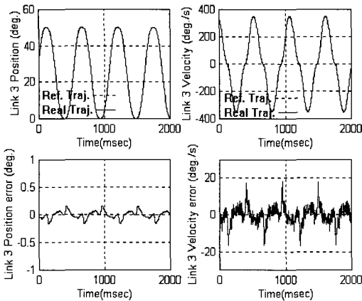
그림 20. PID제어기에 의한 링크3의 위치 및 속도 궤적 추종 결과.
