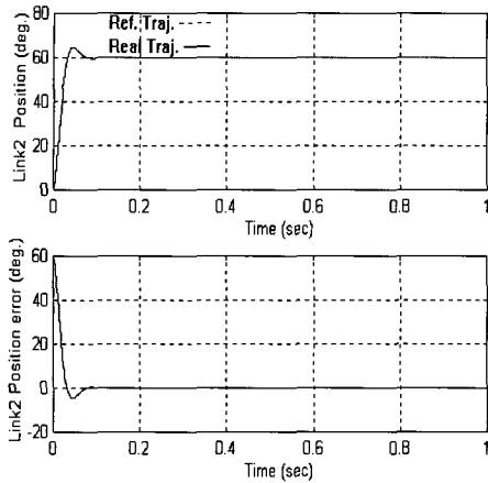
그림 6. 링크2의 위치궤적 추종 결과. Fig. 6. Simulation results of position trajectory tracking for link 2.(4kg payload).
