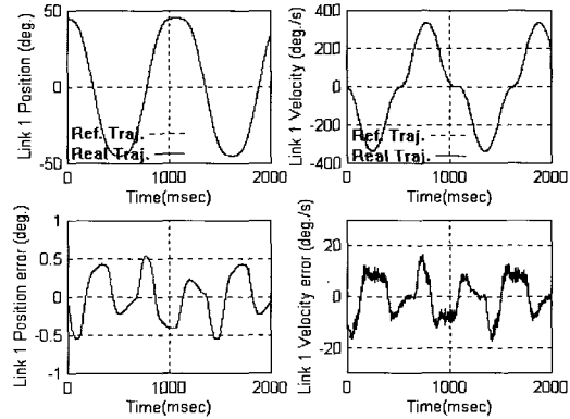
그림 18. PID제어기에 의한 링크1의 위치 및 속도 궤적 추종 결과. Fig. 18. The experimental results of PID controller for position and velocity trajectory tracking of link 1.(2.0kg payload).
