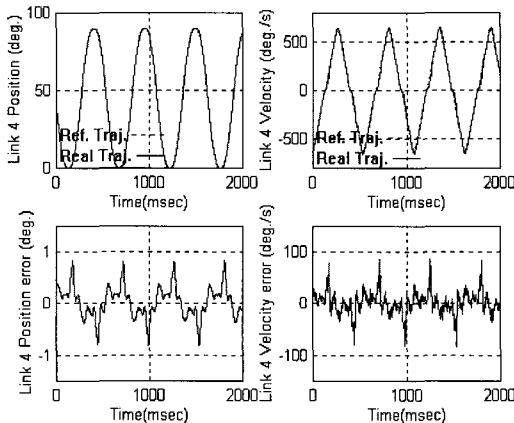
그림 21. PID제어기에 의한 링크4의 위치 및 속도 궤적 추종 결과.
