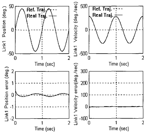
그림 7. 링크1의 위치와 속도 궤적 추종 결과. Fig. 7. Simulation results of position and velocity trajectory tracking for link 1.(2kg payload).
