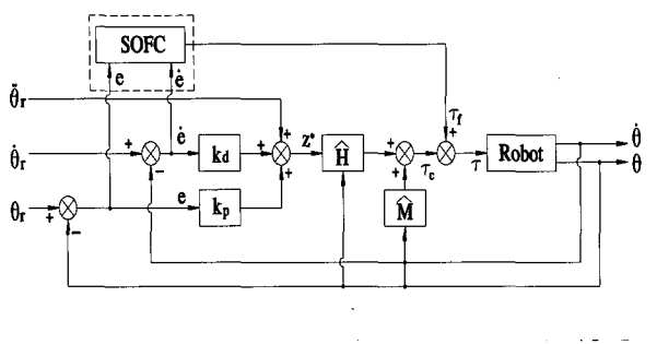
그림 2. 제안된 퍼지제어의 구성도.
