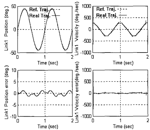
그림 10. 링크2의 위치와 속도 궤적 추종 결과. Fig. 10. Simulation results of position and velocity trajectory tracking for link 2.(2kg payload).
