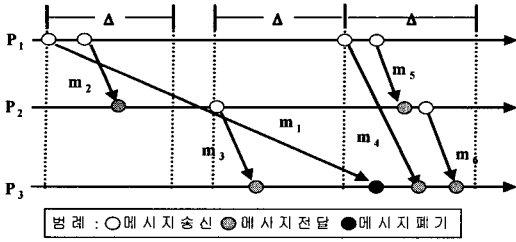
(그림 1) \Delta -인과순서와 인과순서 메시지 전달
