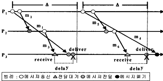
(그림 2) \Delta -인과순서에 따른 메시지 전달
