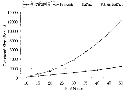
(그림 4) 전송되는 제어정보의 크기 비교
