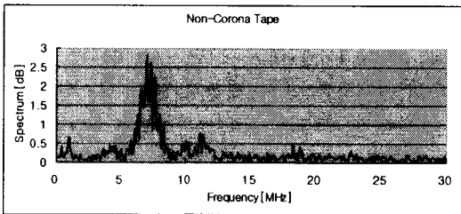
(b)주파수 분석
