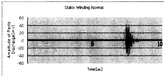
(a)신호파형
