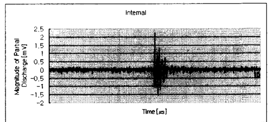
(a) 신호파형
