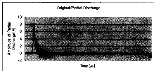
(a)부분방전 원형신호
