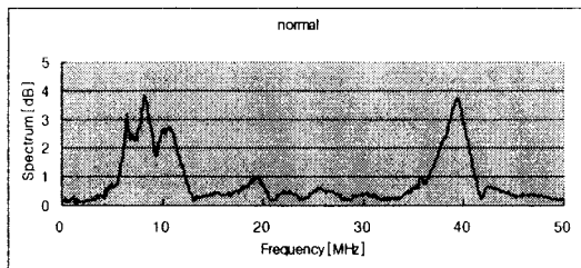
(b)주파수 분석
