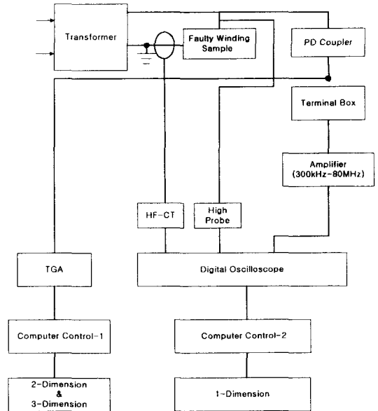
(그림 1) 부분방전 계측시스템 구현
