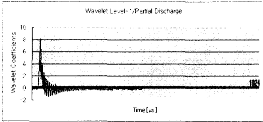
(b)이산웨이블렛 변환 Level-1 (SK=2.34 , KU=5.17) (그림 6) 부분방전신호에의 적용
