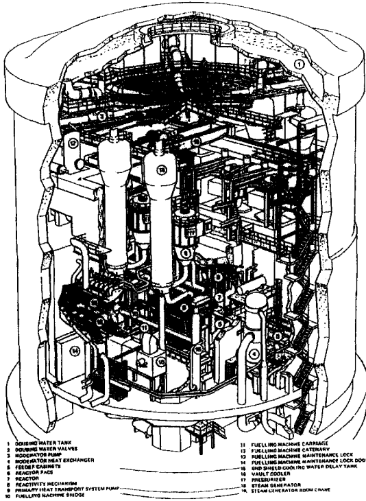
그림 2 월성 2호기 격납건물의 형상 (12)
