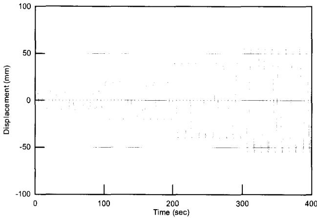
그림 9 특성시험을 위한 수평하중의 변위-시간이력
