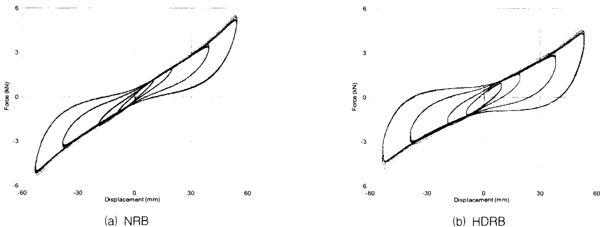
그림 10 고무베어링의 수평전단시험에 의한 하중-변위 곡선
