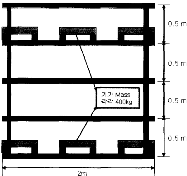
그림 3 실험모형의 제원
