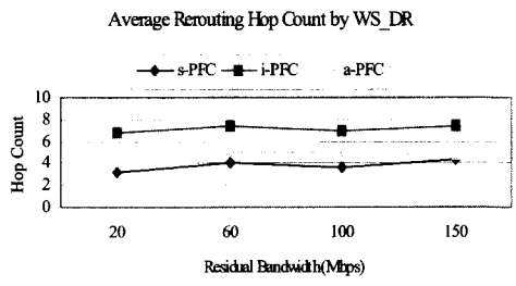
그림 6. WS_DR기법을 이용한 다양한 장애복구 기법 (s-PFC, i-PFC, a-PFC)에 대한 재라우팅 평균 홉수 비교
