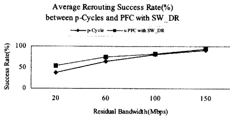
그림 7. SW_DR기법을 이용한 p-Cycle과 s-PFC 기법간의 재라우팅 서비스 성공률 비교
