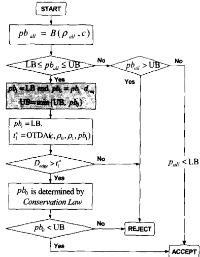
그림 7. 서비스 차등률을 고려한 연결 수락 제어 알고리즘 Fig. 7. Connection admission control algorithm considering service differentiation-ratio
