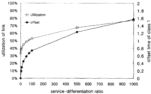
그림 12. 최대 링크 이용률과 extra-offset 시간 Fig. 12. Maximum link utilization and extra-offset time
