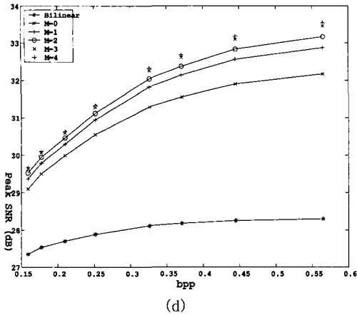
그림 4. JPEG 부호화기의 입력으로 (a) Lena, (b) Watch, (c) Cap, (d) F-16 영상을 이용하였다. JPEG으로 압축된 상태에서 DCT 크기를 변화시켰을 때, 그리고 DCT 크기를 고정시키고 압축률을 변화시켰을 때 PSNR 값을 구하였다. 4 \times 2^{M+1} 크기 DCT 블록을 4 \times 2^M 크기 DCT 블록으로 근사화 하는 방법으로 영상을 가로 세로 각각 반으로 줄인다. 그 후, 4 \times 2^M 크기 DCT 블록을 4 \times 2^{M+1} 크기 DCT 블록으로 근사화 하는 방법으로 영상을 가로 세로 각각 두 배로 늘인다. 여기서 M=0,1,\dots,4 .
