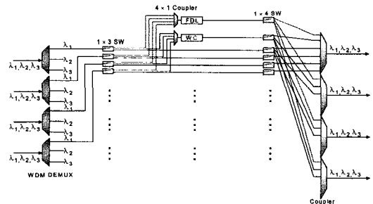
그림 2. 광 버스트 스위치 구조
