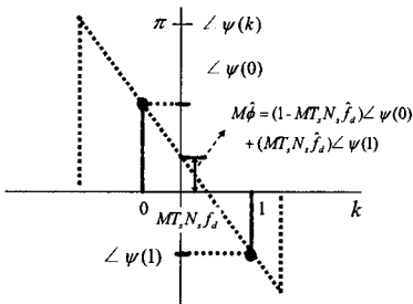
그림 6. 양수의 소수배 주파수 오프셋에서 위상 스펙트럼의 주엽과 상관값의 스펙트럼 및 첫번째 LJE
