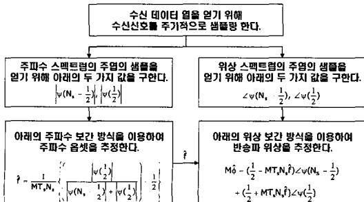
그림 10. 제안된 두 번째 LJE의 절차 흐름도
