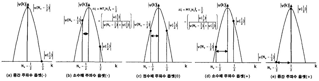
그림 8. 다양한 주파수 오프셋에 따른 주파수 스펙트럼의 주엽과 상관값의 스펙트럼 및 제안된 두 번째 LJEА
