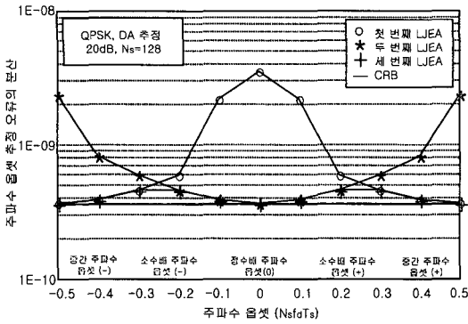
그림 7. 정규화 된 주파수 오프셋에 따른 DA 주파수 오프셋 추정 성능의 변화
