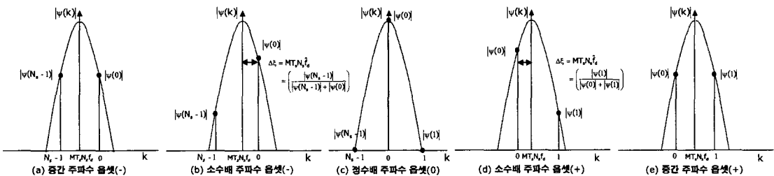
그림 5. 다양한 주파수 음셋에 따른 주파수 스펙트럼의 주엽과 상관값의 스펙트럼 및 제안된 첫 번째 LJEA
