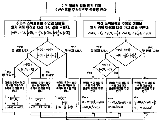
그림 11. 제안된 세 번째 LJEAs의 흐름도
