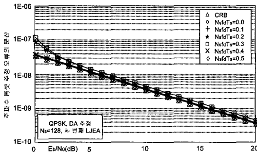
그림 8. E_b/N_0 에 따른 데이터 보조(DA) 주파수오프셋 추정 성능의 변화
