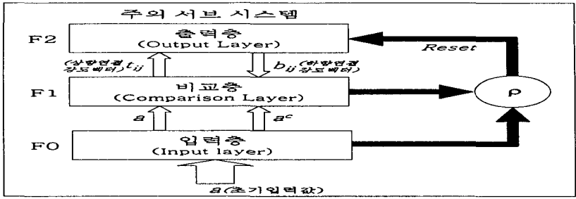
< 그림 1 > Fuzzy ART 신경망의 구조
