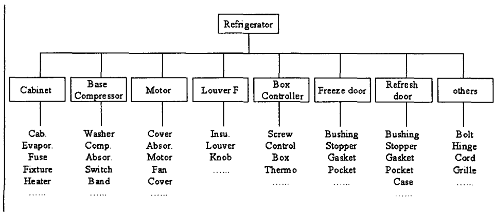
< 그림 2 > 냉장고의 구조
