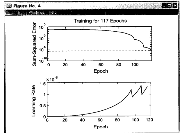
(그림 8) 뉴런 수가 12인 경우
