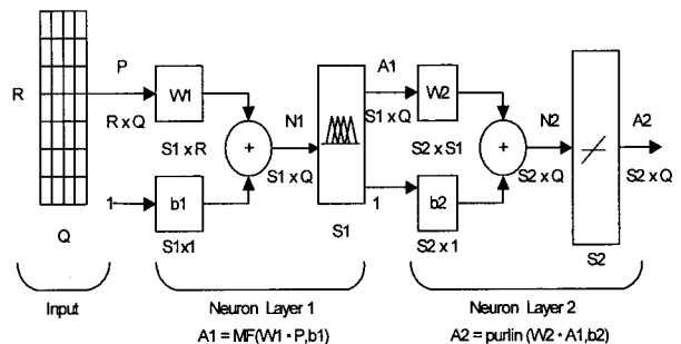
(그림 5) 퍼지 멤버십 함수와 신경망의 소프트웨어 모델
