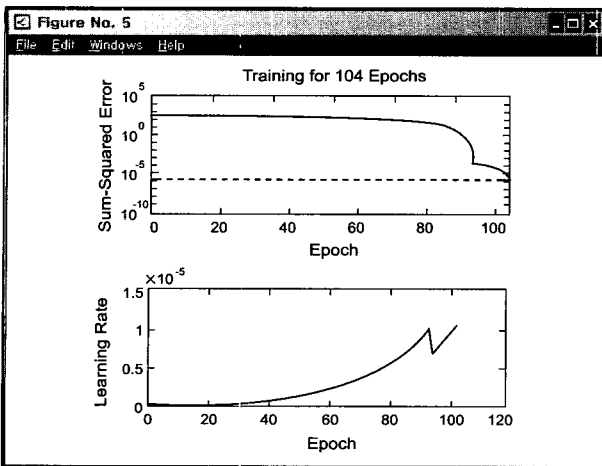
(그림 9) 뉴런 수가 15인 경우
