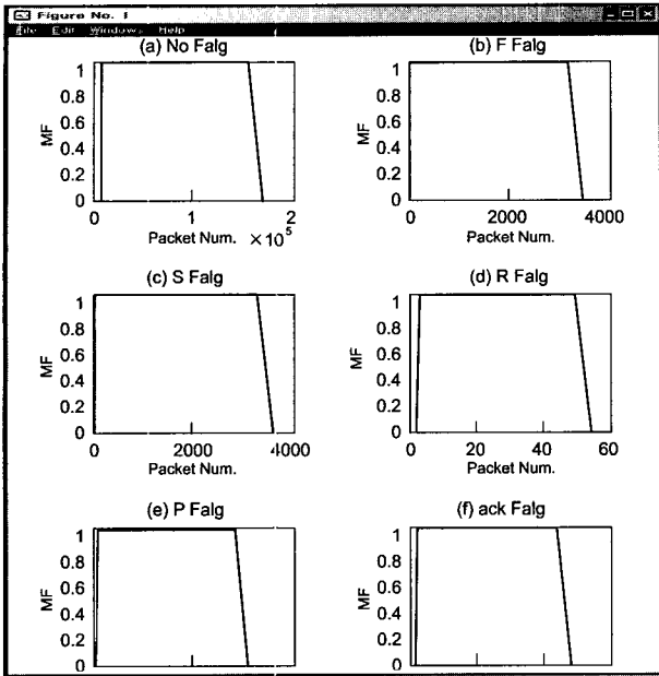
(그림 4) 플래그별 사다리꼴 멤버십 함수
