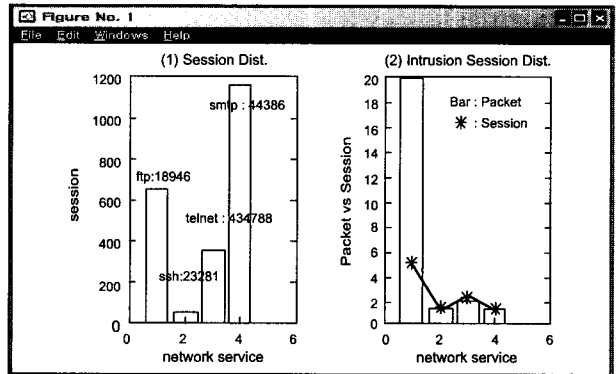
(그림 10) 정상과 침입의 세션 분포
