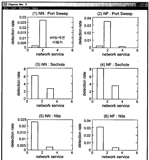
(그림 11) 신경망과 뉴로-퍼지에 의한 침입 탐지 결과
