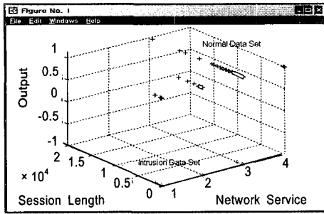
(그림 12) 정상 데이터와 침입 데이터의 분포
