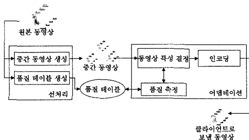
그림 8 준-동적 어댑테이션 모델
