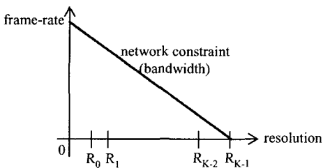
그림 11 네트워크 제약, 해상도, 프레임 율 관계
