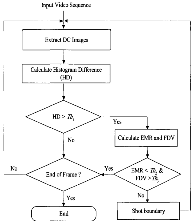
그림 1. 제안한 알고리즘의 흐름도. Fig. 1. Flowchart of the proposed algorithm.
