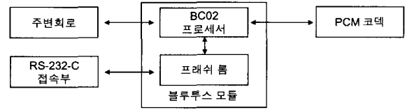
(그림 2-2) 설계된 시스템의 하드웨어 환경
