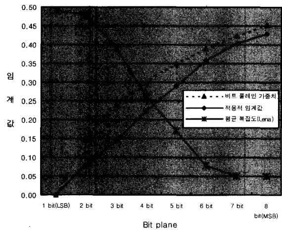
(그림 5) 복잡도와 가중치를 이용한 적응적 임계값 (Lena, block size = 2^3 \times 2^3 , k = 0.15 )
