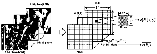
(그림 8) 비트 플레인과 2^m \times 2^m 크기의 블록
