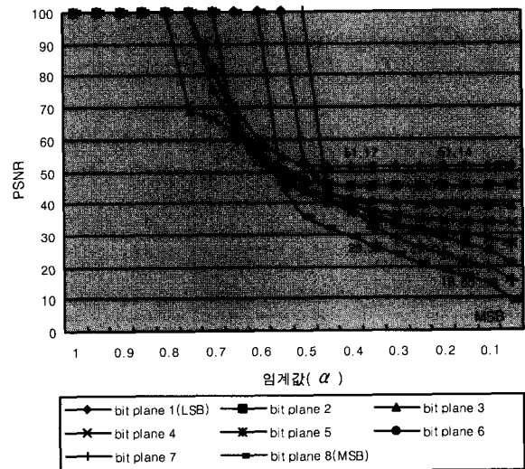
(b) 임계값에 따른 비트플레인별 화질 변화
