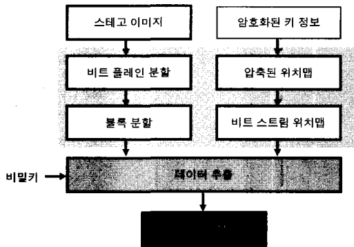
(그림 9) 추출 알고리즘의 블록도
