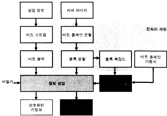
(그림 6) 삽입 알고리즘의 블록도
