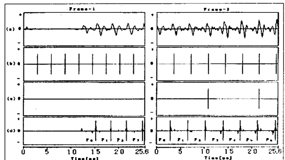
그림1. 피치추출 (a) 원음성 (b) 자기상관법 (c)Cepstrum법 (d)개별피치 추출법
