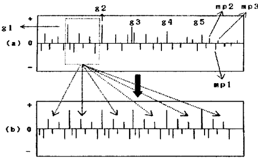
그림2. 멀티펄스의 진폭과 위치
