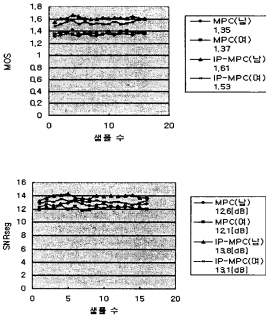
그림4. SNRseg와 MOS Fig.4 SNRseg and MOS
