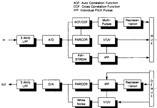
그림3. IP-MPC 방식의 블록도 Fig.3 Block diagram of IP-MPC
