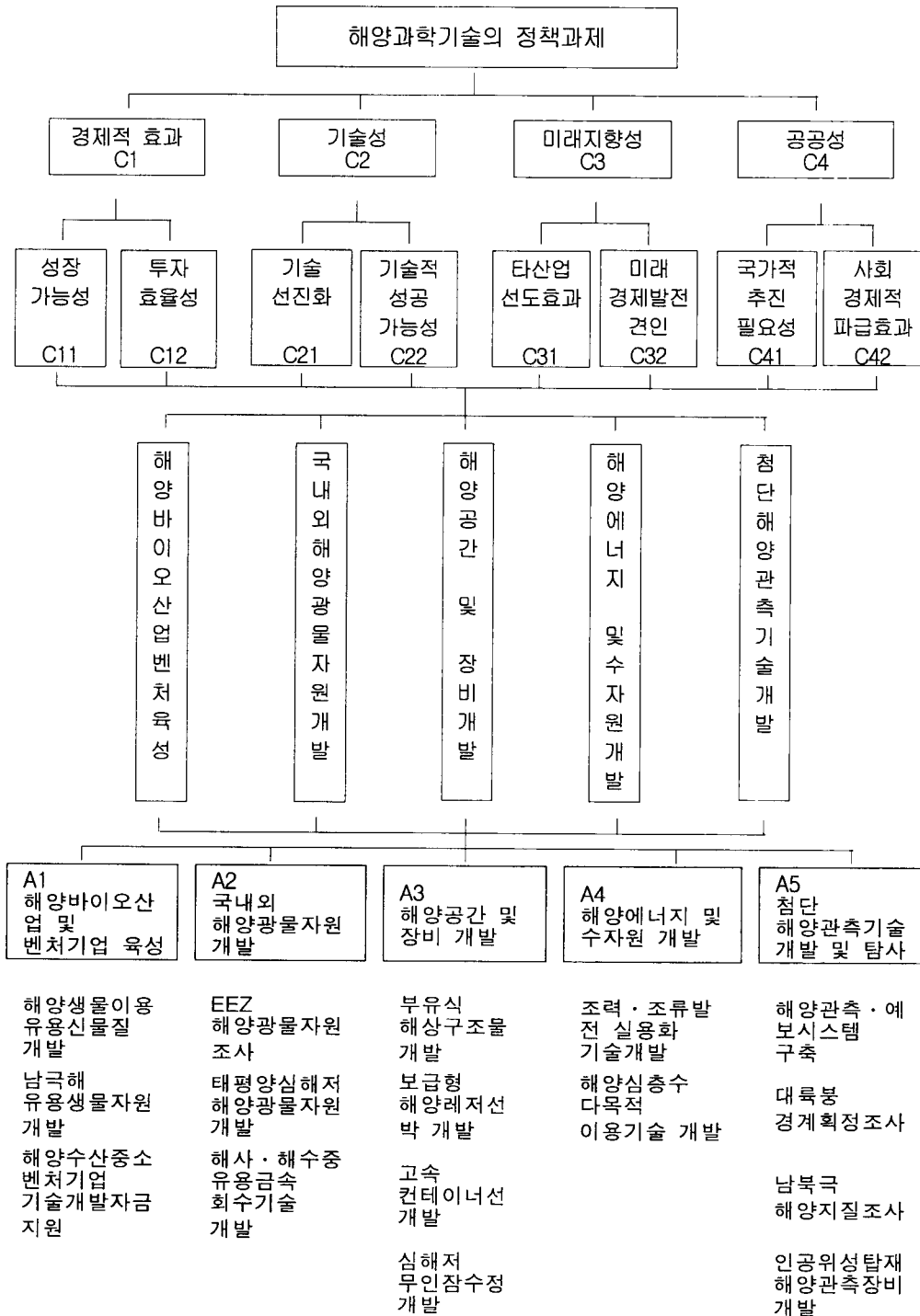
<그림 1> 해양과학기술개발 분야의 계층구조
