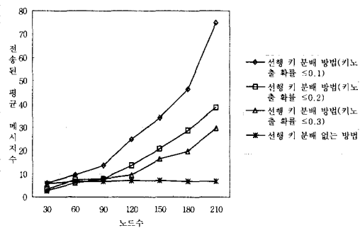
그림 5. 노드수의 증가에 따른 평균 전송 메시지
