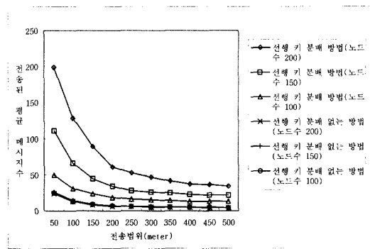
그림 4. 전송범위의 증가에 따른 평균 전송 메시지
