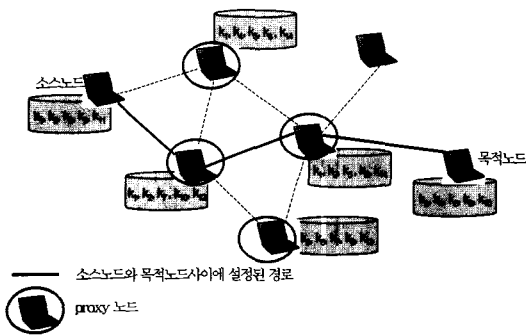
그림 1. 확률적인 키 공유 기반의 단 대 단 키 설정 방법 서 동작할 수 있다.
