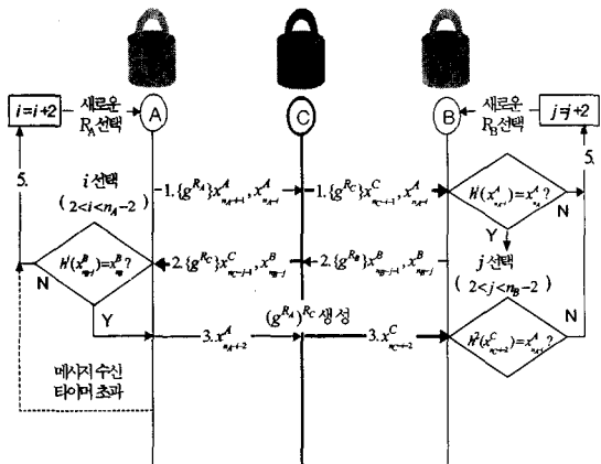
그림 3. 단대 단 키 설정에 대한 man-in-the-middle 공격
