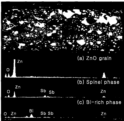
그림 2. 시편 A의 EDAX 패턴.
