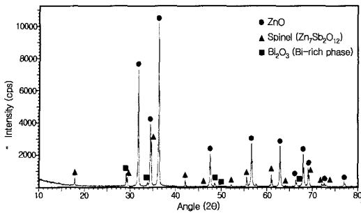
그림 1. 시편 A의 X선 회절 패턴.
