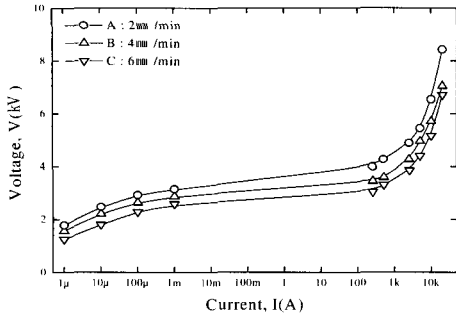
그림 3. 소성조건에 따른 각 소자의 전압(V)-전류(I) 특성 곡선.
