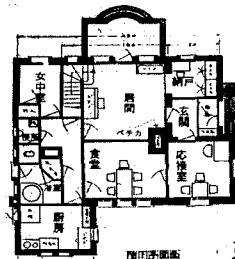
그림 4. 3등 2석 1층 평면도
