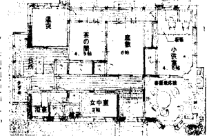
그림 2. 2등 평면도
