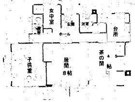
그림 10. 2등2석 평면도
