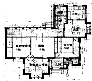
그림 3. 3등 1석 평면도
