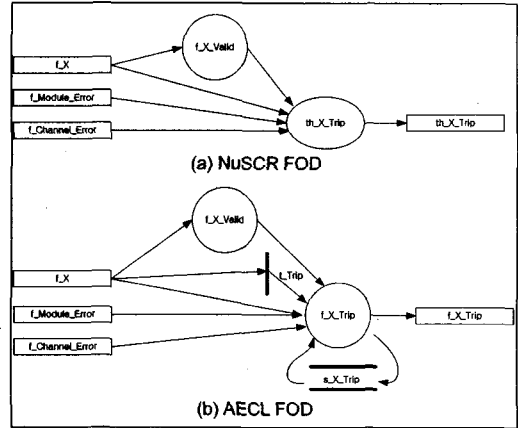
그림 1 Simplified FOD for g\_SGI\_LVL\_Lo\_RPS
