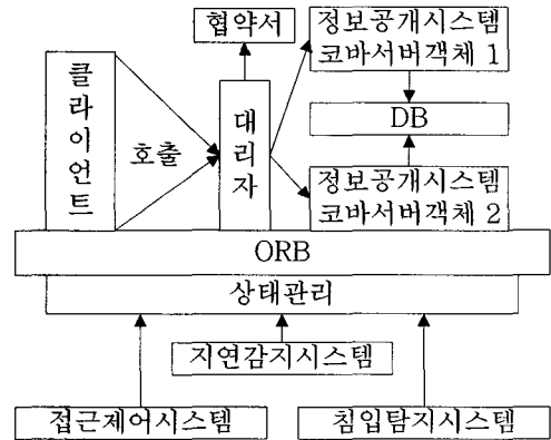
그림 14. 침입감내응용시스템
