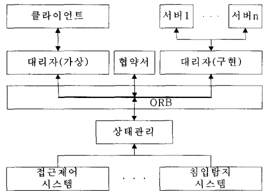
그림 6. 침입감내시스템의 응용아키텍처
