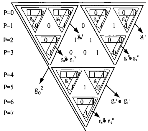
그림 10. 3변수에 대한 삼각 셀 방법 적용 예. Fig. 10. An Example using Triangle cell for 3-variable.
