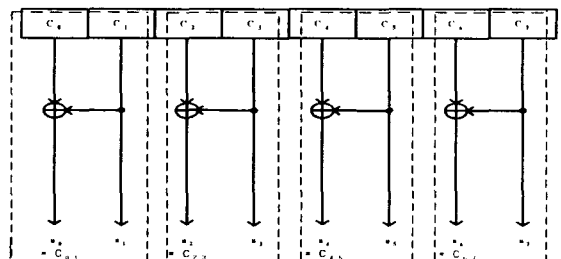
그림 3. 단일변수에 대한 기본적인 변환 회로.
