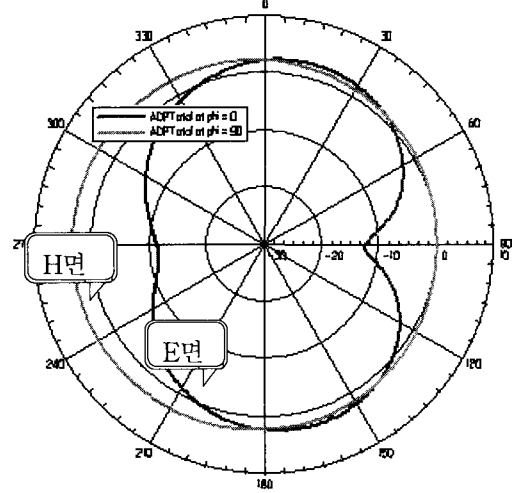
그림 11. Chip Antenna의 방사패턴(E면,H면) Fig. 11 Radation pattern of chip antenna (E-Plane, H-Plane)
