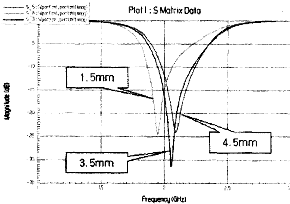
그림 5. 급전 위치 변화에 따른 공진주파수 특성 Fig. 5. Resonant frequency characteristic versus change of feed line position
