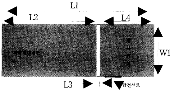
그림 3. 단순화된 chip antenna 아래면 구조 Fig. 3. Under plane of simplified chip antenna
