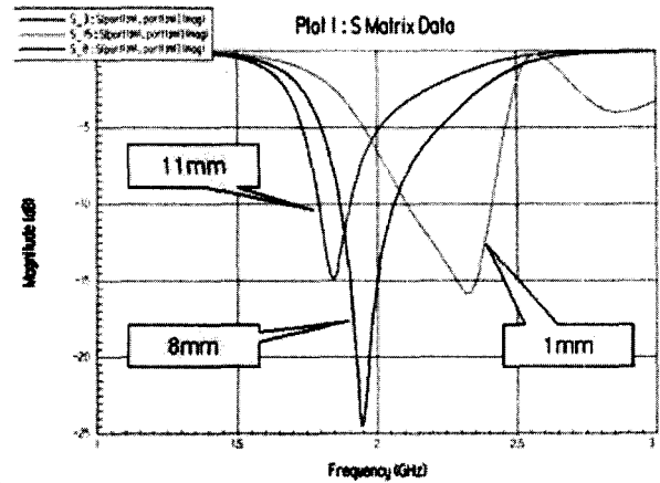
그림 10. 용량의 위치 변화에 따른 공진주파수 특성 Fig. 10. Resonant frequency characteristic versus change of capacitor position
