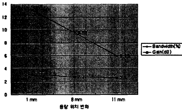
그림 9. 용량의 위치 변화에 따른 이득과 대역폭 Fig. 9. The gain and bandwidth versus change of capacitor position
