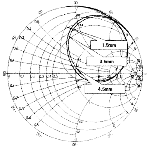
그림 6. 급전점의 위치 변화에 따른 입력 임피던스 특성 Fig. 6. Input Impedance characteristic versus change of feed line position
