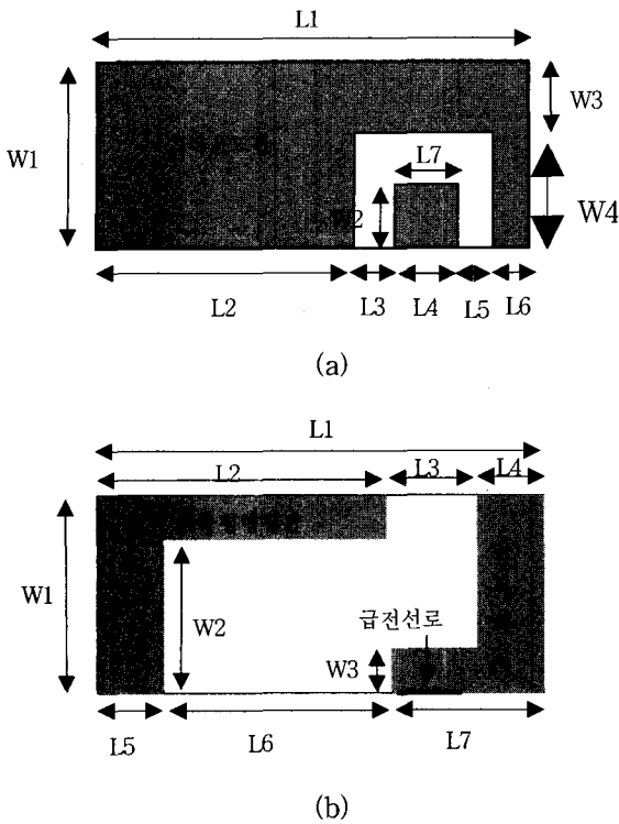
그림 1. Chip Antenna 구조 (a) 윗면 (b) 아랫면
