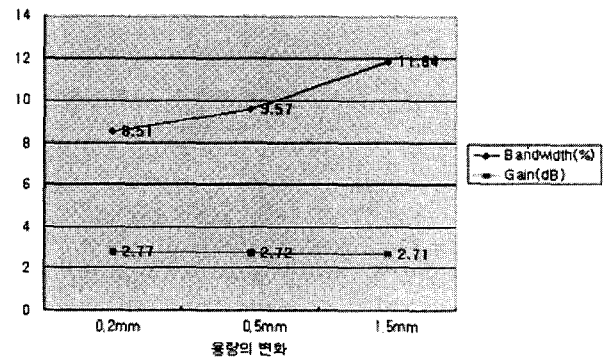
그림 7. 용량의 변화에 따른 이득과 대역폭 Fig. 7. The gain and bandwidth versus change of capacitor
