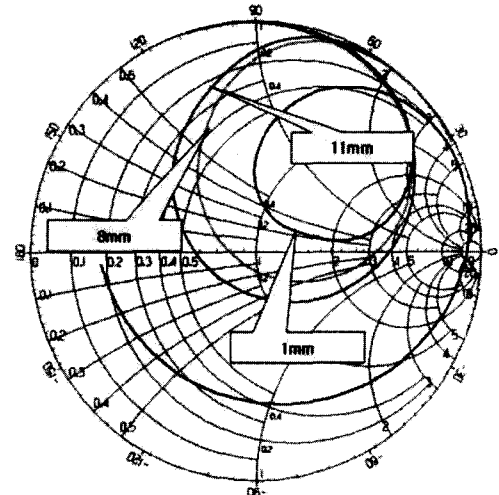
그림 11. 용량의 위치 변화에 따른 입력 임피던스 특성 Fig. 11. Input impedance characteristic versus change of capacitor position
