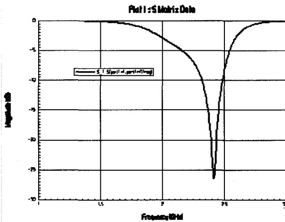
그림 12. Chip Antenna의 리턴로스 특성 Fig. 12 Return loss characteristic of chip antenna
