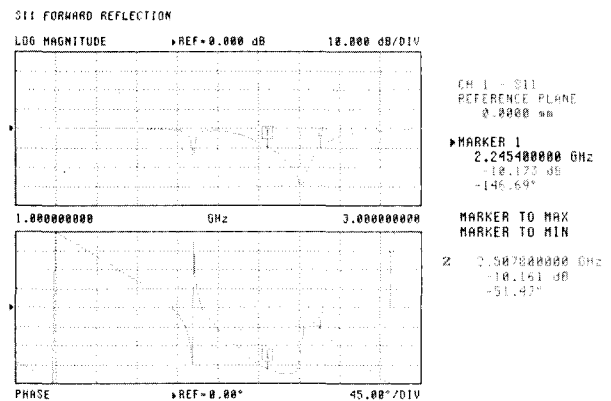
그림 13. 측정된 Chip 안테나의 리턴로스와 위상 Fig. 13 The Return loss and phase of measured chip antenna
