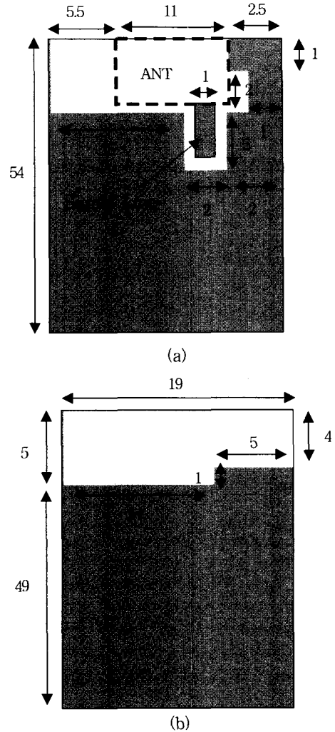
그림 2. Bluetooth PCB Layout (a) 윗면 (b) 아랫면
