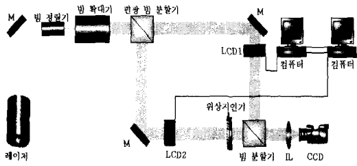
그림 2. 복소 홀로그램의 실시간적 복원 시스템도
