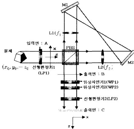
그림 1. 변형된 삼각 간섭계 시스템도
