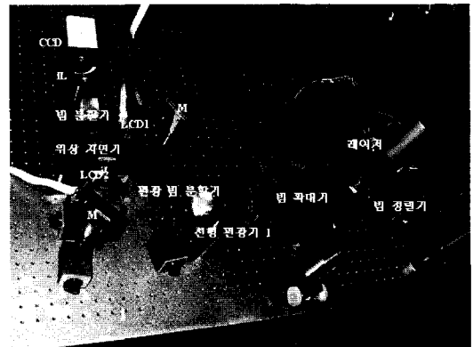
그림 4. 합성된 복소 홀로그램의 복원을 위한 광학 시스템도
