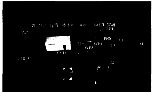
그림 8. 인코히어런트 복소 홀로그래ム 합성을 위한 광학계
