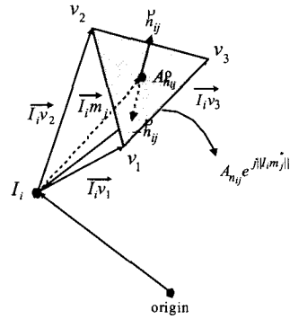
그림 4. i 번째 패치 P_i 로 분류된 j 번째 메쉬의 법선 벡터 \vec{n}_{ij}^* ( -\vec{n}_{ij} ) 및 CEGI의 복소 가중치.
