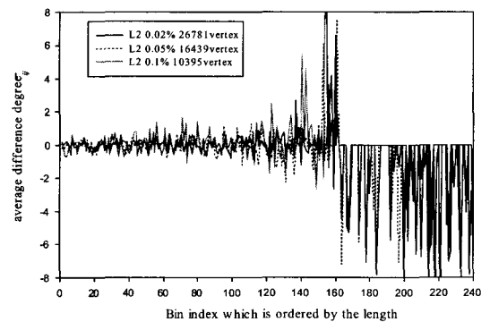
그림 8. Stanford Bunny 모델의 첫 번째 패치에서 각 셀의 평균 법선 벡터 방향 \bar{\theta} 과 메쉬 간단화 공격된 모델에 대한 각 셀의 평균 법선 벡터 방향 \bar{\theta}' 와의 차이.
