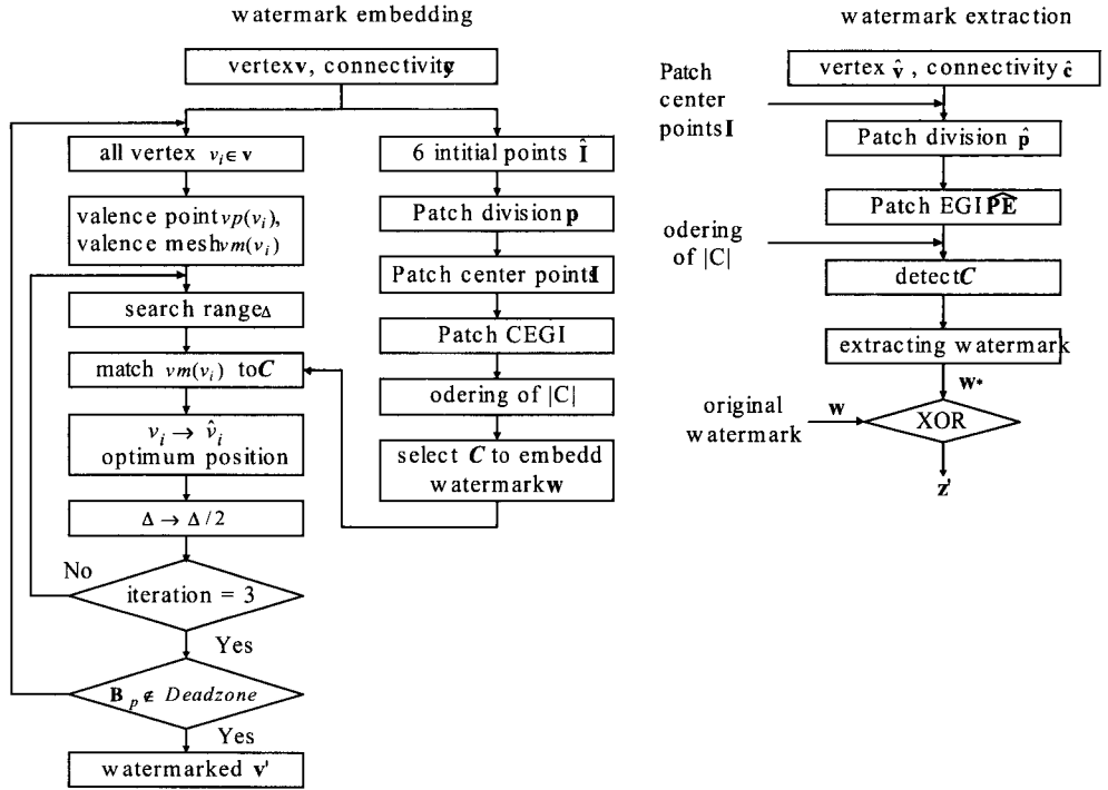
그림 2. 제안한 알고리즘의 워터마크 삽입 및 추출 블록도.
