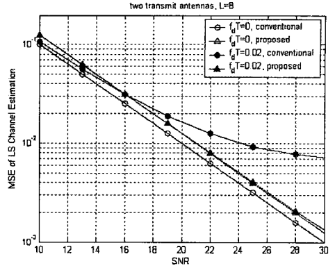
그림 3. 채널 변화에 따른 각각의 채널 추정 방법의 MSE 성능 비교
