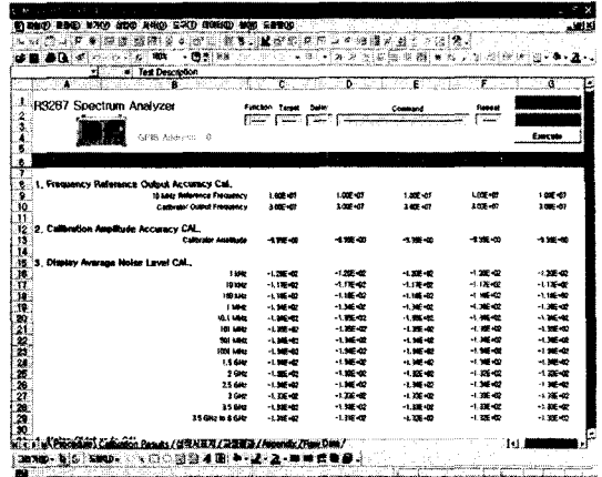
그림 4.3 Spectrum Analyzer의 교정 결과
