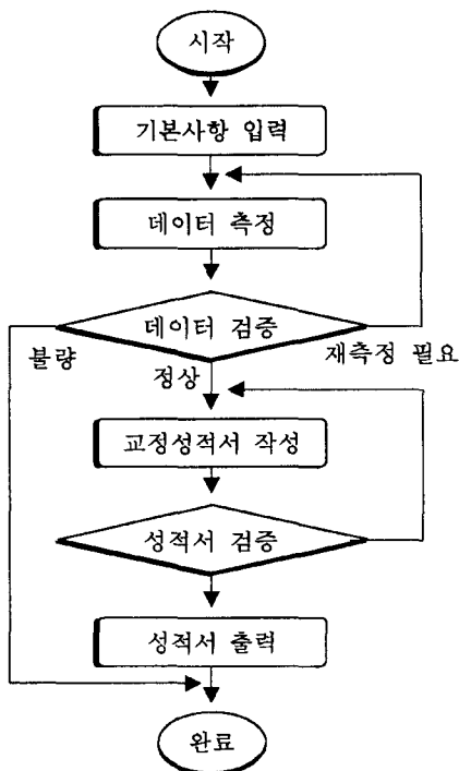
그림 3.1 Calibration Process
