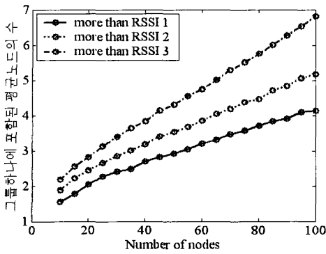
그림 12. 깊이우선탐색에서의 그룹화 결과 그룹하나에 포함되는 평균 단말개수.
