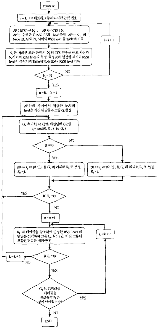
그림 4. 제안된 깊이우선탐색을 이용한 중계 단말 선정 및 단말그룹 알고리즘.
