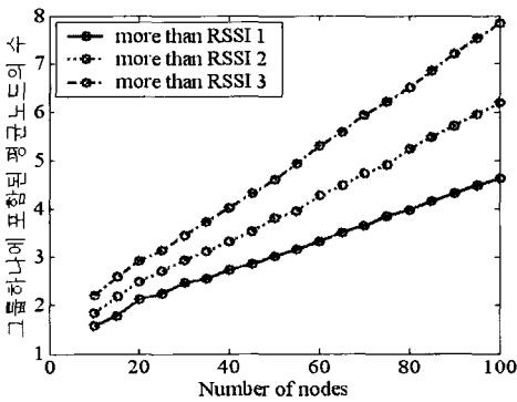
그림 13. 넓이우선탐색에서의 그룹화 결과 그룹하나에 포함되는 평균 단말개수.
