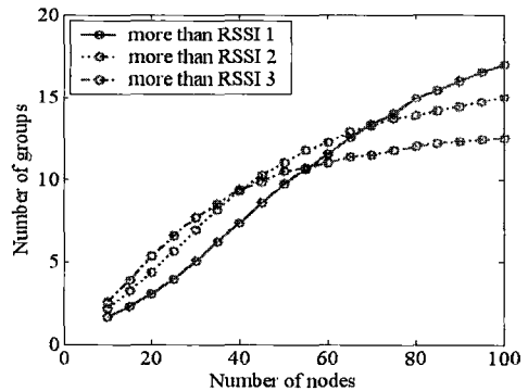
그림 10. 깊이우선탐색결과 생성되는 그룹개수.
