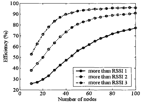
그림 14. 깊이우선탐색에서의 그룹화 효율.
