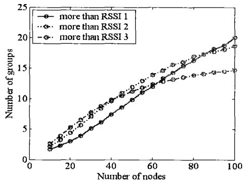
그림 11. 넓이우선탐색결과 생성되는 그룹개수.
