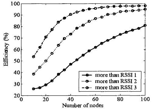
그림 15. 넓이우선탐색에서의 그룹화 효율.
