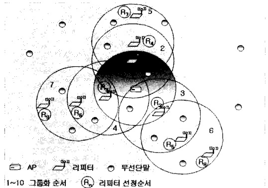
그림 6. 넓이우선탐색에 의한 그룹화의 예.
