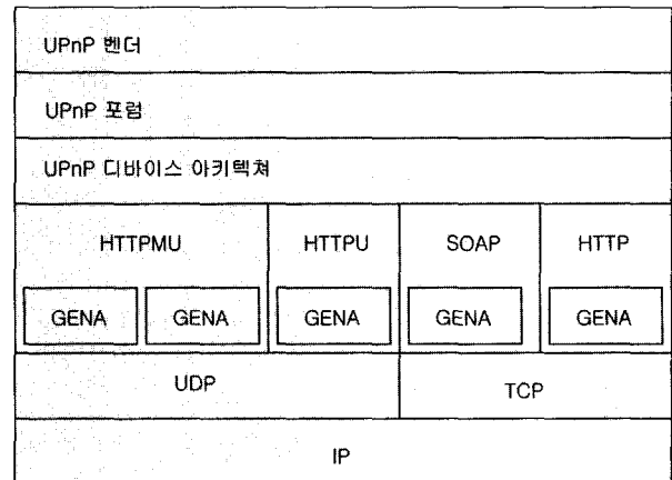
(그림 1) UPnP 프로토콜 스택
