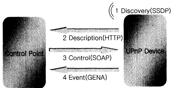
(그림 2) UPnP 동작과정
