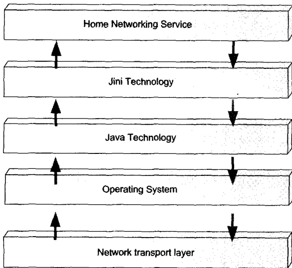
(그림 4) Jini 소프트웨어 구조
